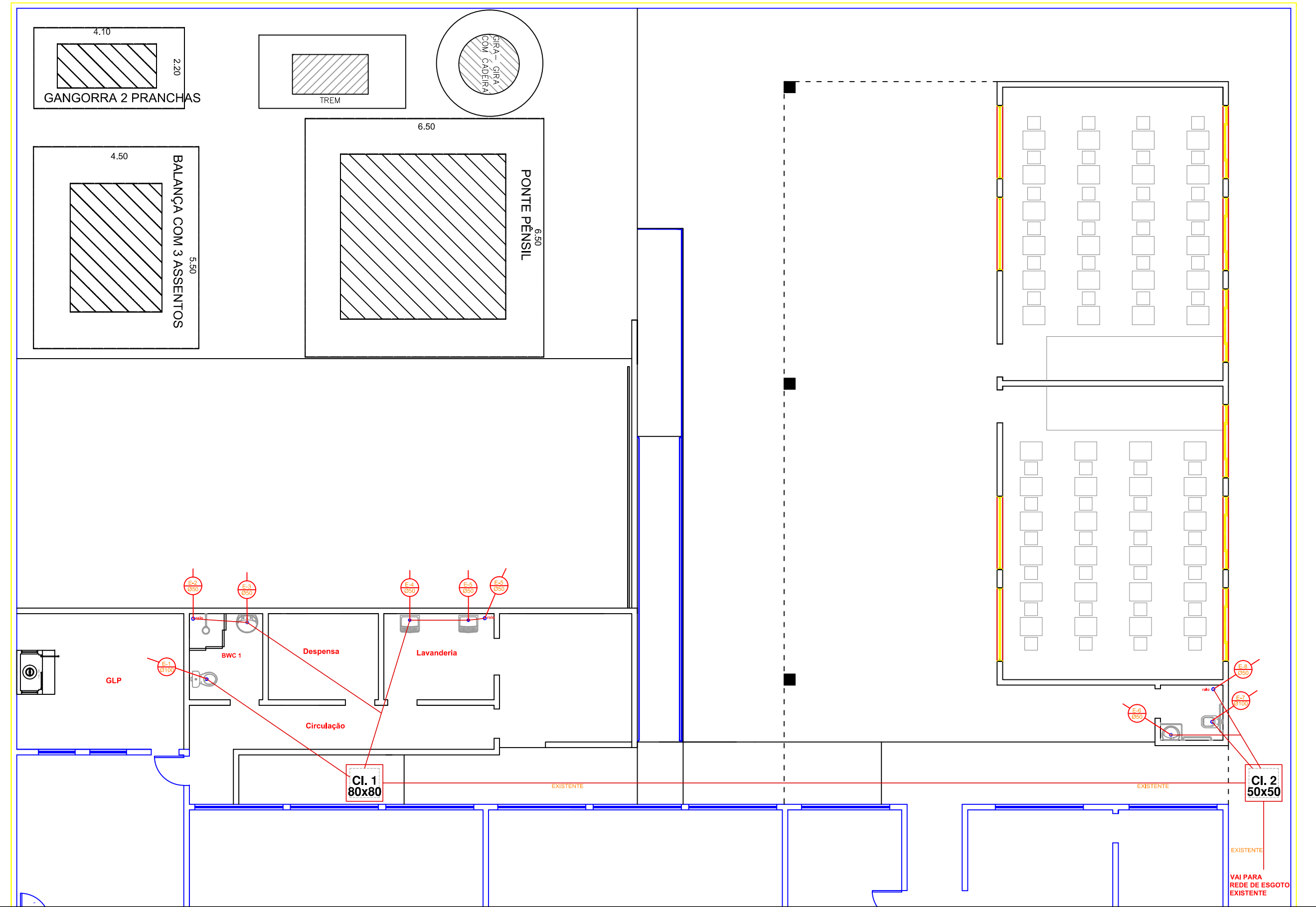
PLANTA BAIXA SANITÁRIO Esc. 1:100
