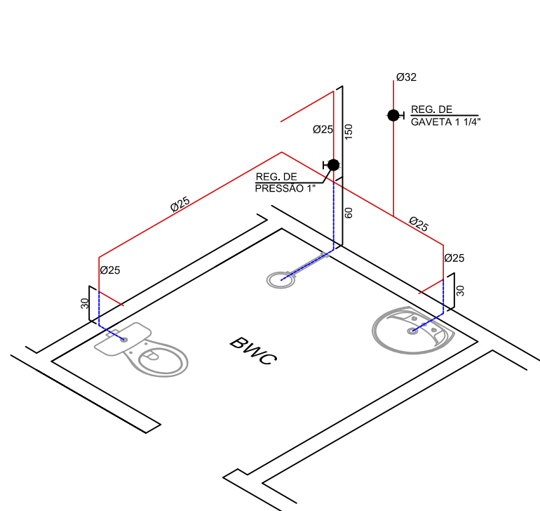
DET.ISOM-1 ESCALA: 1:20
