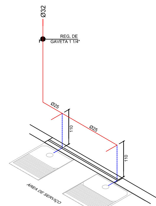
DET.ISOM-2 ESCALA: 1:20
