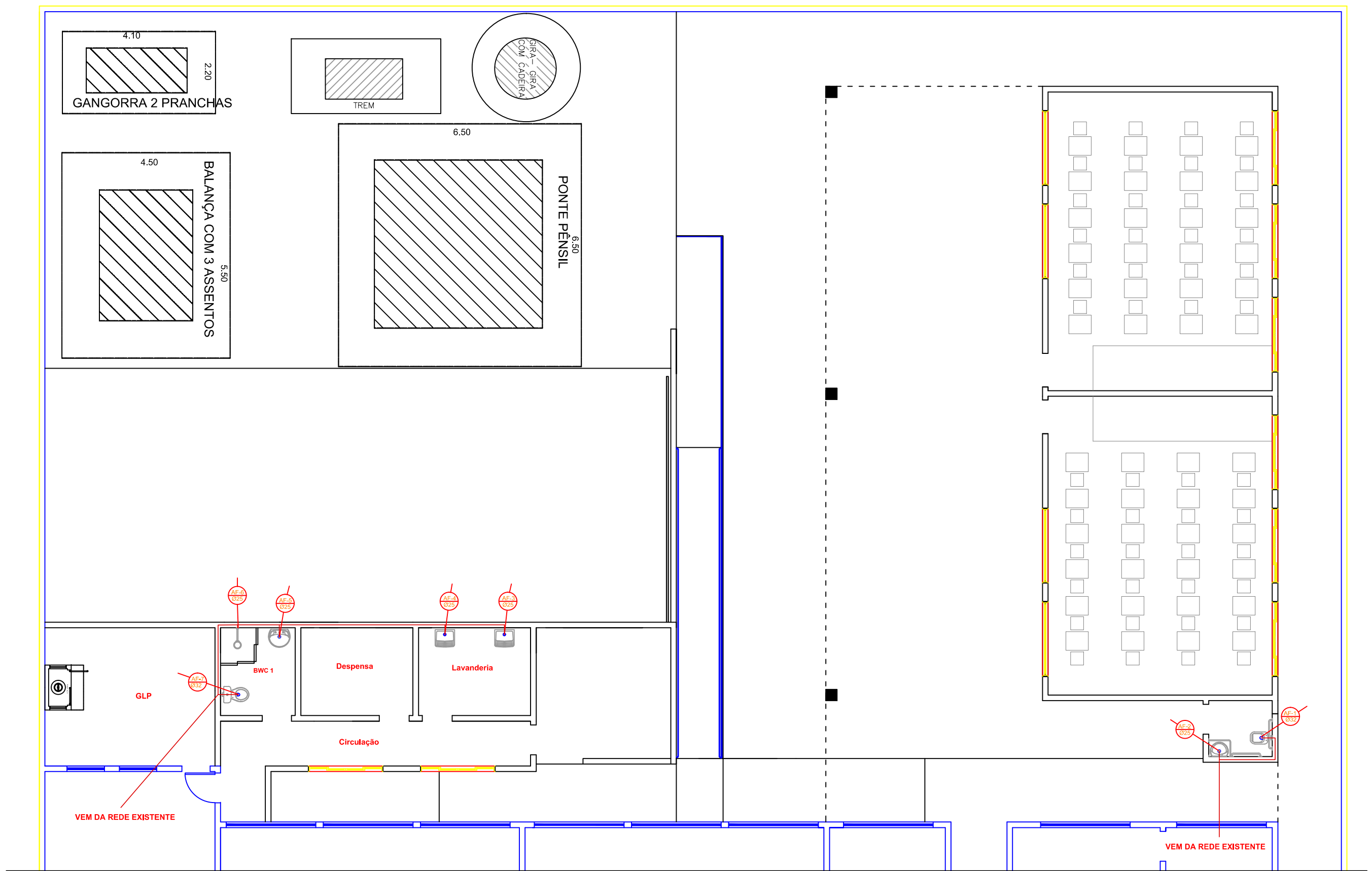
PLANTA BAIXA HIDRAULICO Esc. 1:100
